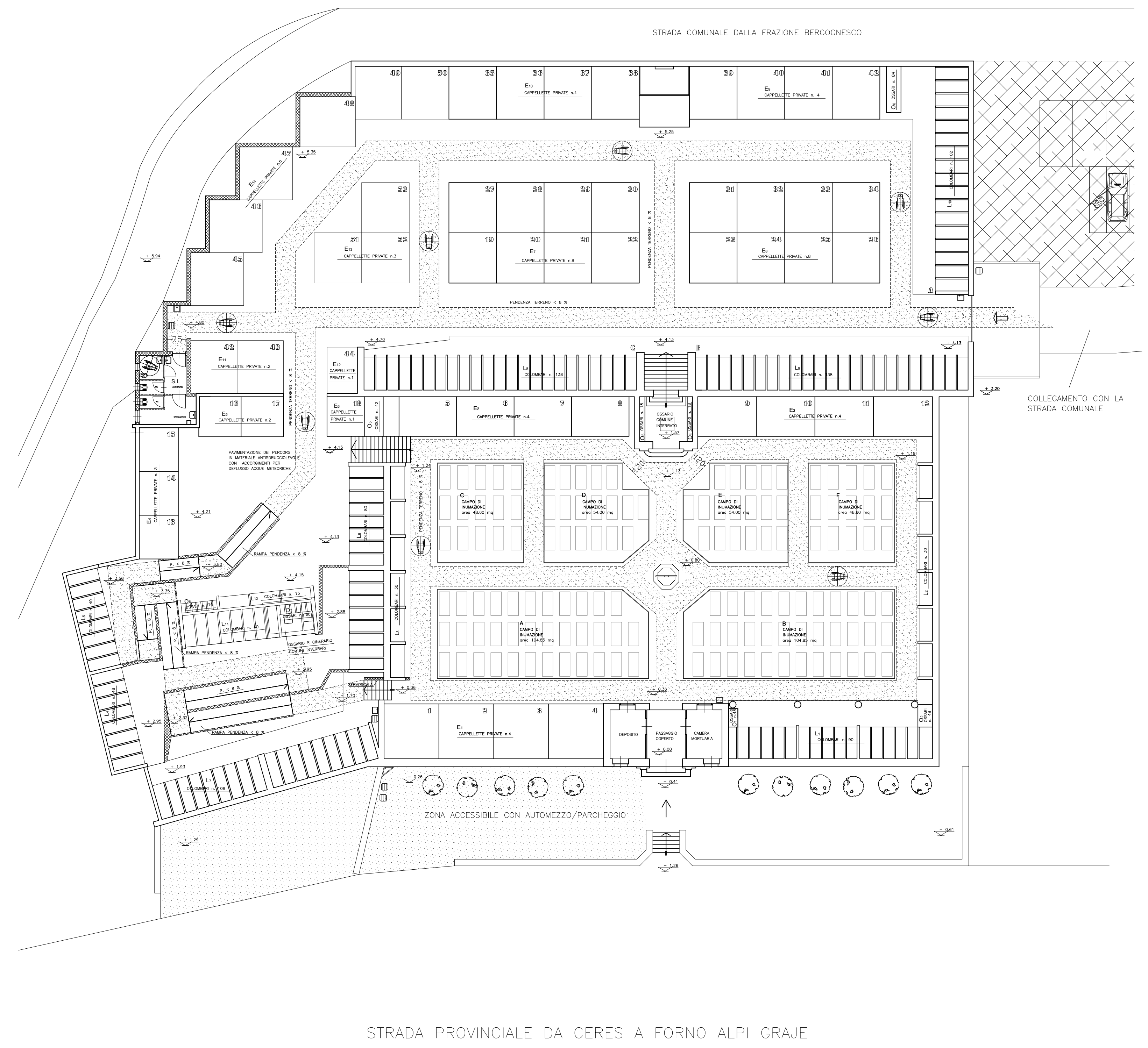
PLANIMETRIA GENERALE – PREVISIONI Scala 1: 200
